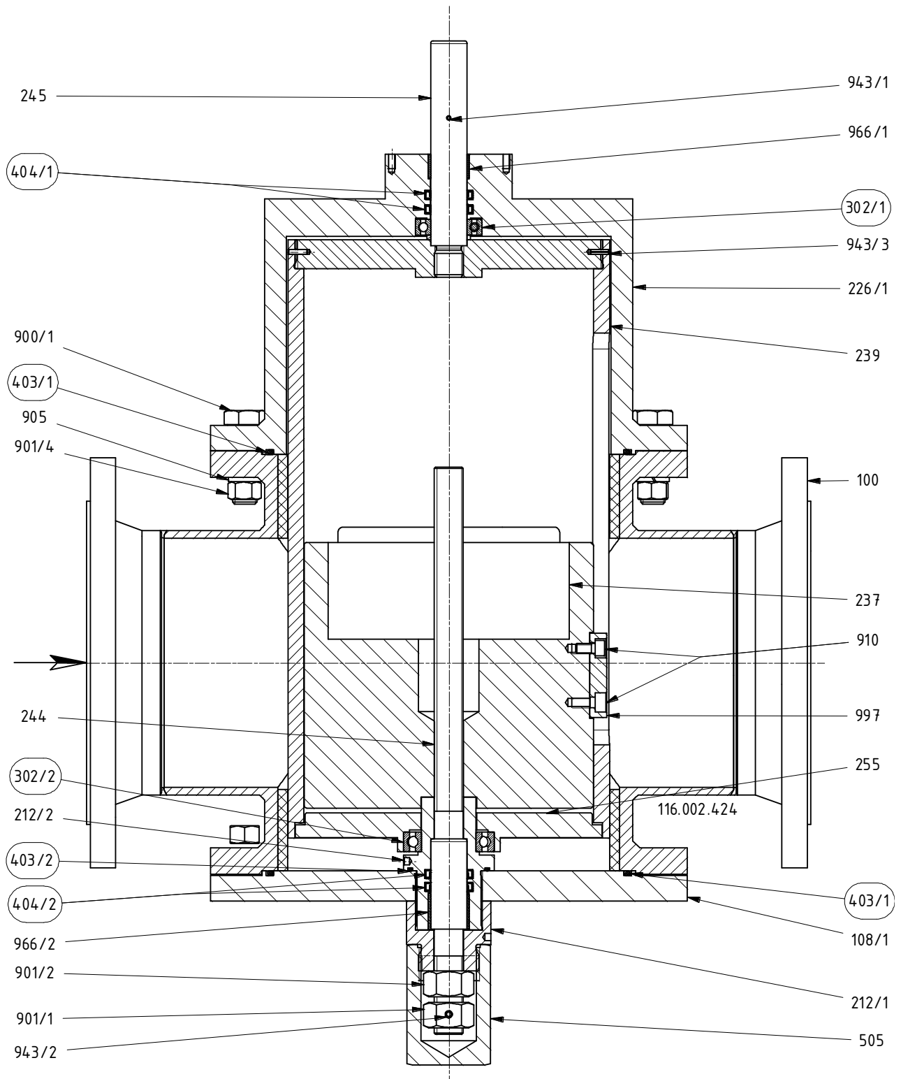
Abb.3 Schnittzeichnung DN 200
